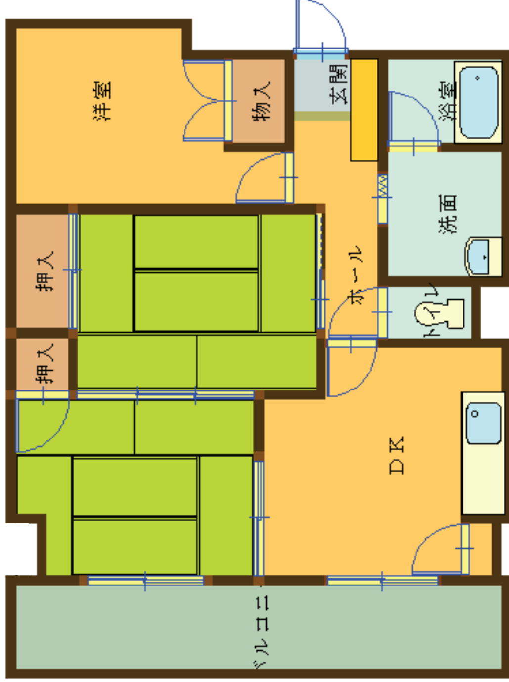
医師官舎の間取り (3DK) (台所・和室6畳2室・洋室5.5畳)
